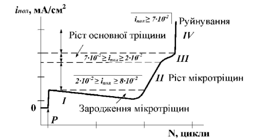
Критичні значення густини струму поляризації сталі 08X18H10T на різних ступенях її пошкодження. I–IV – періоди руйнування.
