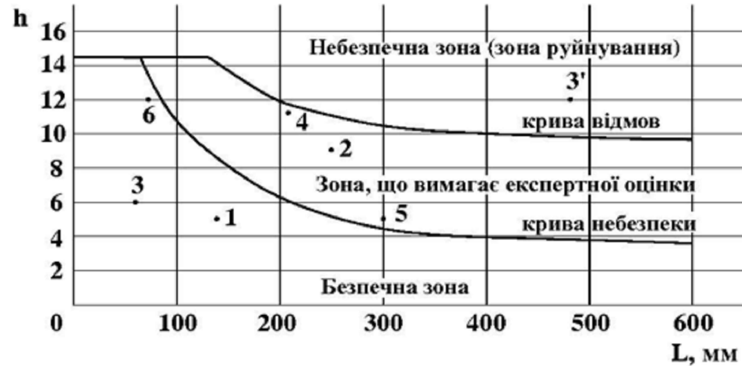
“Критерій В31G” із стандарту ANSI/ASME B31 G-1984
