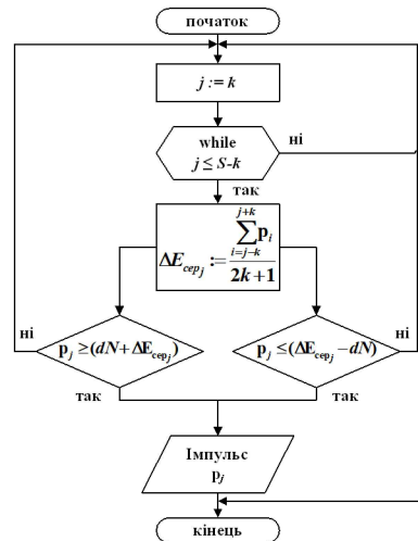
Структурна схема алгоритму ідентифікації електрохімічних імпульсів.
