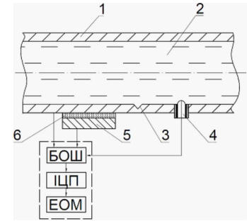
Загальна схема конструкції датчика.
