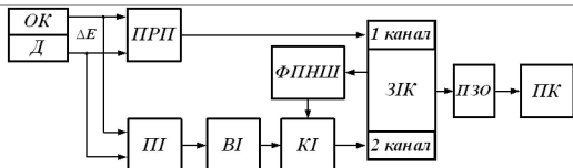
Структурна схема ЕІМ на основі аналогової ідентифікації імпульсів руйнування:
